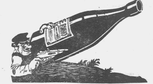
Томе „готовятся“
