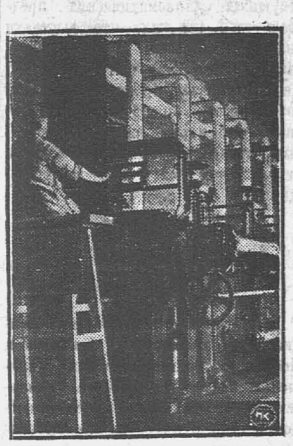
На снимке—Первый Экземпляр сконструированного и изготовленного Путиловским заводом аппарата для обработки и промывки тканей после крашения. Установлен на ситце-печатной фабрике им. Свердлова в Москве. До сих пор такие аппараты ввозились из-за границы.
