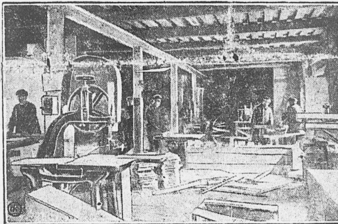
На снимке: внутренний вид механической части дереводоблочной мастерской.
