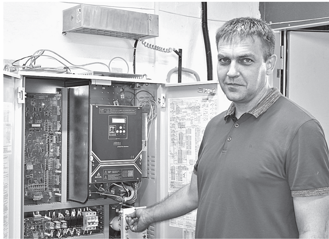
Александр Благодатских показывает, как работает станция управления.
