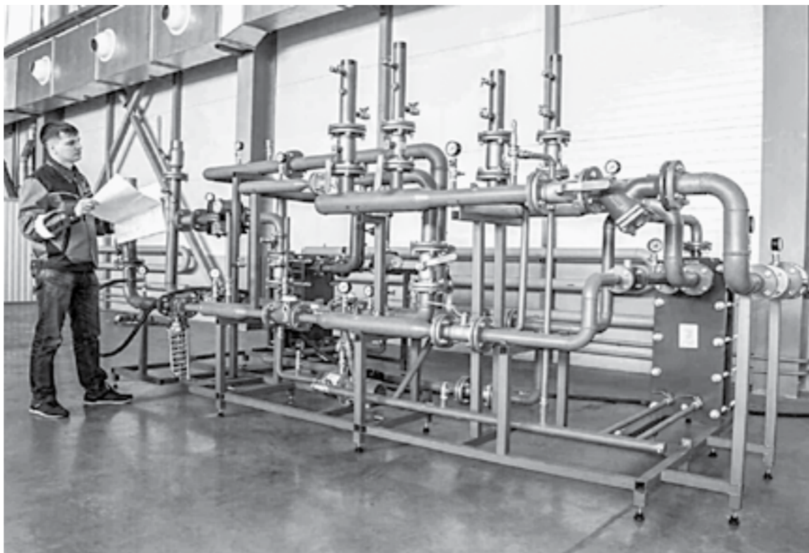
Так выглядит индивидуальный тепловой пункт.
