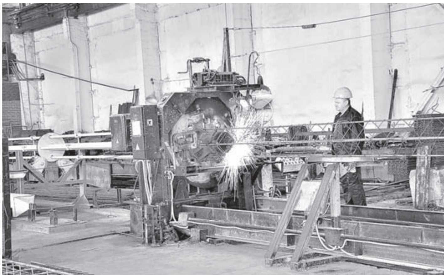
Сварочный станок по изготовлению арматурного каркаса для свай.
