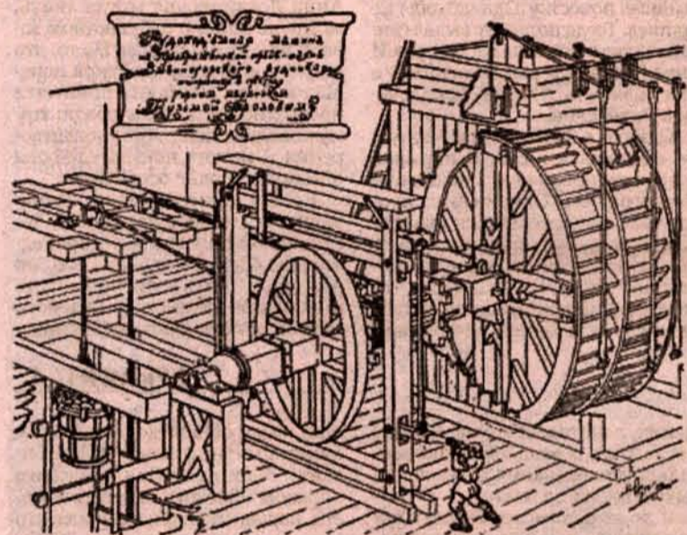
Чертеж рудоподъёмной машины в Змеиногорске.
