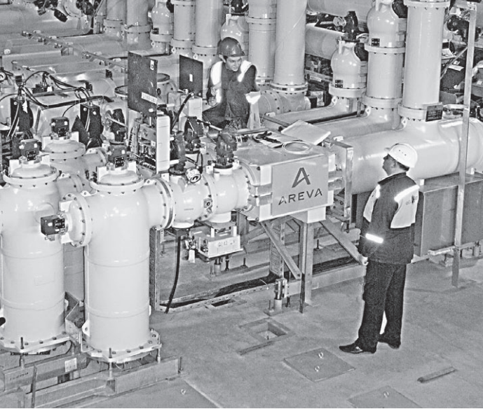
Конструкция на переднем плане, возле которой стоит Вадим Кравченко, и есть то самое КРУЭ французского производства. А сверху его «соседа» электромонтажник из Томска Дмитрий Карачев. Старый советский образец устройства занимал примерно половину видимой на фото площади да еще под открытым небом.
