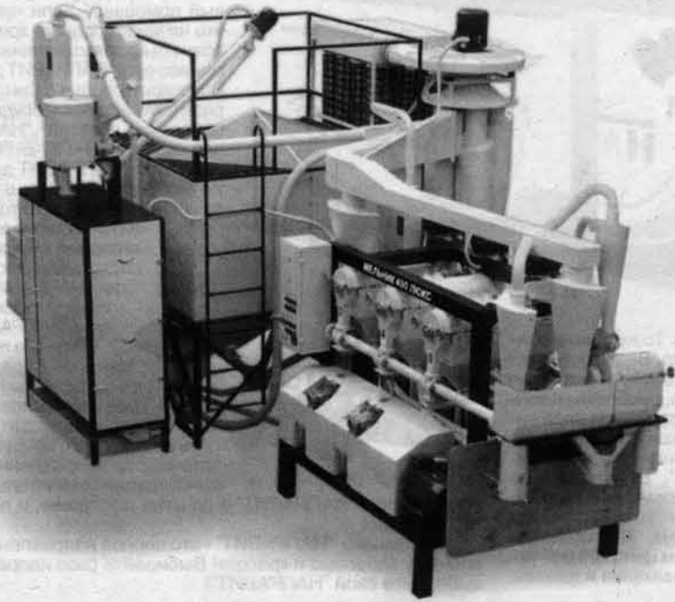
МЕЛЬНИК 400 ЛЮКС (производительность мельницы 400 кг зерна в час, выход 37% муки высшего сорта и 37% муки первого сорта).
