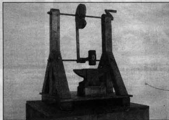
Механическая наковальня.
