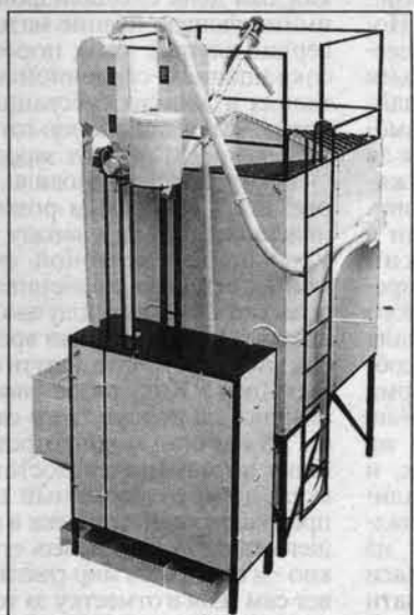
Мощная система очистки, увлажнения и отволаживания зерна - гарант получения прекрасной муки на мельницах "Мельник".
