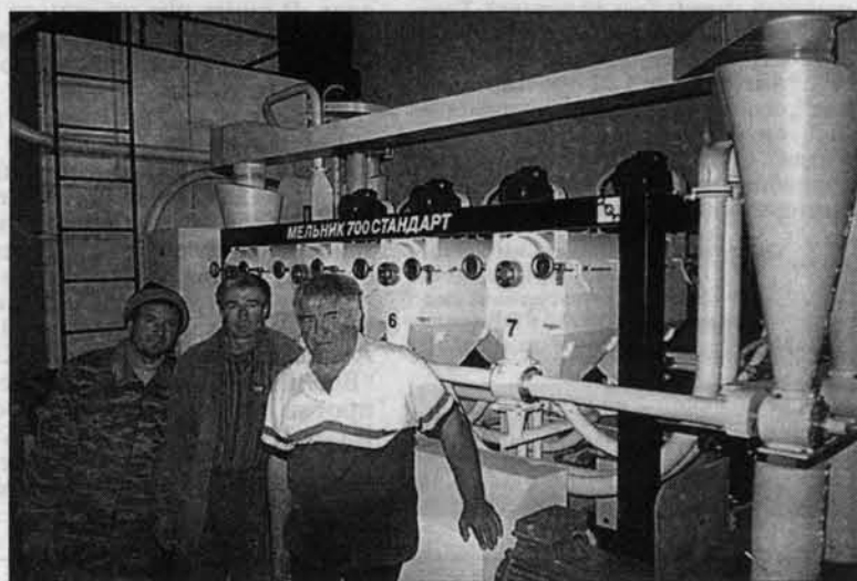
Мельница "Мельник 700 стандарт" (село Чумашки, Новосибирская область). Хозяева довольны высоким качеством муки и экономным потреблением электричества.
