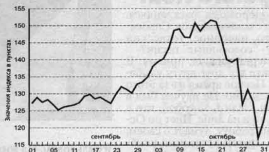
Динамика сводного фондового индекса S&P/RUX в сентябре – октябре 2003 г.
