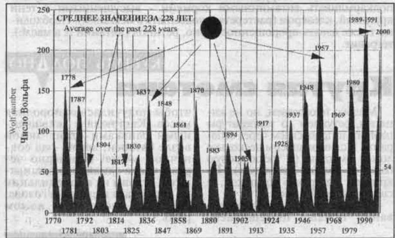
Динамика солнечной активности (число Вольфа) за период 1770-2000 гг.
