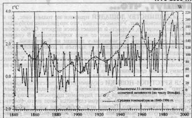
Среднегодовые температуры воздуха (г. Барнаул, 1840-2000 гг.)
