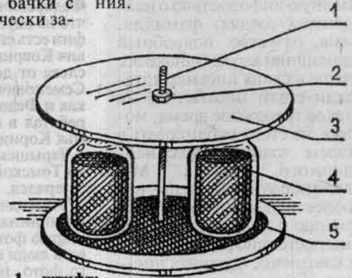
1 - штифт; 2 - гайка; 3 - металлический диск (3-5 мм); 4 - банка с мясом; 5 - резиновая прокладка.
