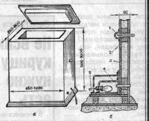
«Погреб» на балконе с откидной крышкой: а - общий вид; б - устройство обогрева; 1 - термометр; 2 - пенопласт; 3 - шлаковата; 4 - крепеж; 5 - электропроводка.
