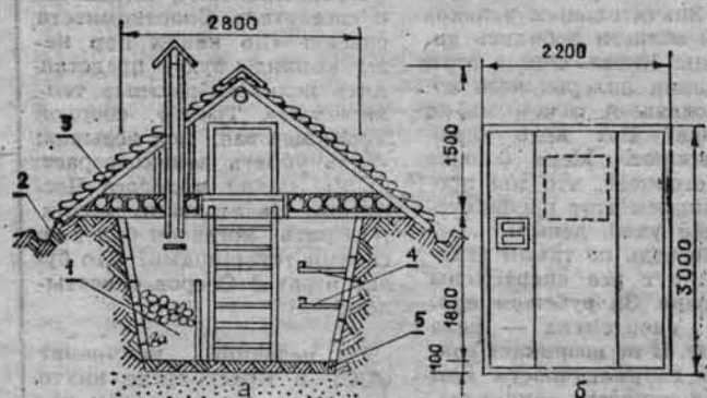
а — Разрез; б — план; 1 — закроем для картофеля; 2 — водоотводная канава; 3 — скат крыши; 4 — полки; 5 — глинобитный пол.
