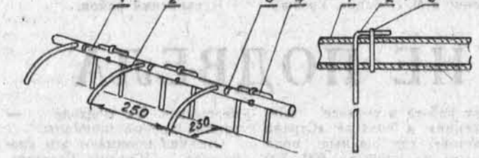
Приспособление Морозова.
