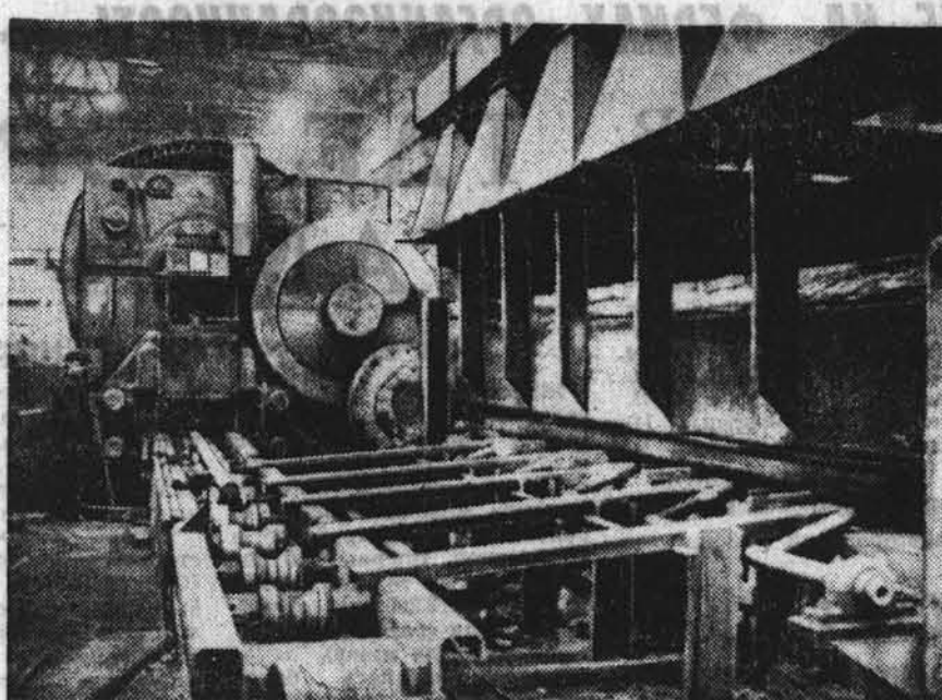
На снимке: на углительном участке кузнечно-прессового цеха АТЗ установлено новое оборудование. Фото В. Колесникова.
