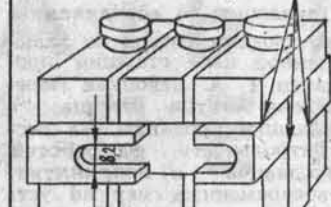
Так, в «Москвиче-2140» эти емкости (чистые банки из-под моторного масла) устанавливаются в карете, укрепленную на кронштейне смятаемого лобового стекла автомобиля. На чертеже представлены эскизы кассеты (точные размеры выверены в соответствии с имеющимися у вас флягами).
