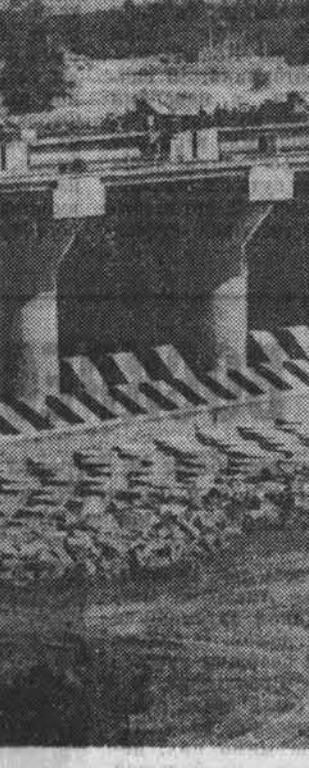
На гидроэнергетическом и навигационном комплексе «Железные ворота-По» на Дунае, сооружаемом совместно Румынией и Югославией, завершены работы по строительству одного из основных объектов ГЭС — водозливной плотины (на снимке).
