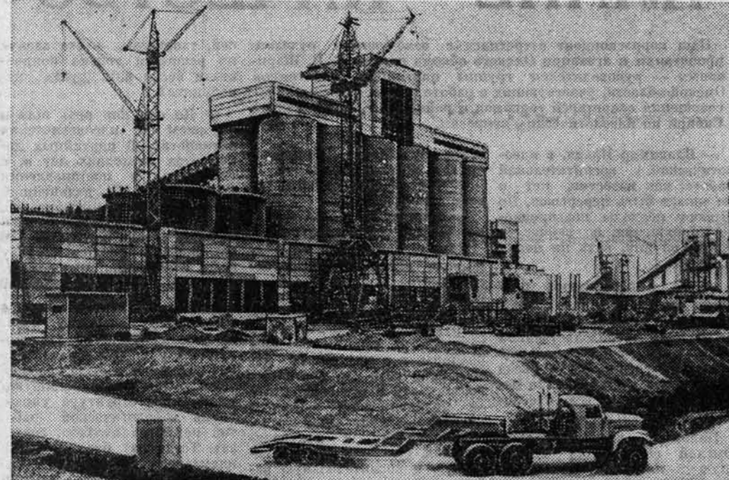
ПЕРВАЯ ОЧЕРЕДЬ АЛТАЙСКОГО КОКСОХИМИЧЕСКОГО ЗАВОДА — ЭТО МНОЖЕСТВО СЛОЖНЫХ ИНЖЕНЕРНЫХ СООРУЖЕНИЙ, РАСКИНУТЫХ НА 160 ГЕКТАРАХ. НА ПРОМЫШЛЕННОМ ПЛОЩАДКЕ УЛОЖЕНО 176 ТЫСЯЧ КУБОВЫХ МЕТРОВ БЕТОНА, СМОНТИРОВАНО 23 ТЫСЯЧИ ТОНН МЕТАЛЛИЧЕСКИХ КОНСТРУКЦИЙ.
