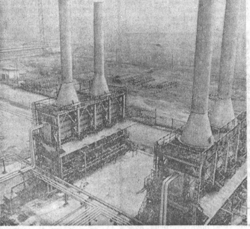
НА СНИМКЕ: новый газоперерабатывающий завод. Фото МТИ—ТАСС.
