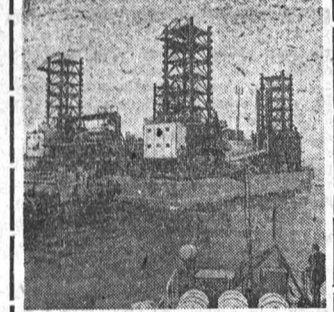
Завершая переход от устья Волги, в станицу Азербайджана приближалась плавучая буровая установка «Ваня» (на снимке). Этот передвижной стальной островок, предназначенный для бурения скважин на участках моря глубиной до 60 метров, построено корабельными мастерами завода «Красные баррикады».
