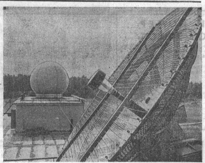
ЦЕНТРАЛЬНАЯ АЭРОЛОГИЧЕСКАЯ ОБСЕРВАТОРИЯ На Центральной аэрологической обсерватории (г. Долгопрудный, Московской области) внедрен новый метод зондирования атмосферы при помощи угольных отражателей. Этот метод позволяет получать достаточно надежные данные о скорости и направлении ветра на разных высотах и в несколько десятков раз снизить затраты на исследования. НА СНИМКЕ: антенны метеорологических радиолокаторов. Фото Б. Корзина. Фотохроника ТАСС.
