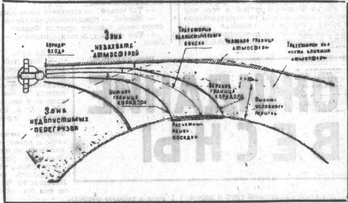
Схема полета автоматической станции «Зонд-5» по трассе Земля—Луна—Земля.
