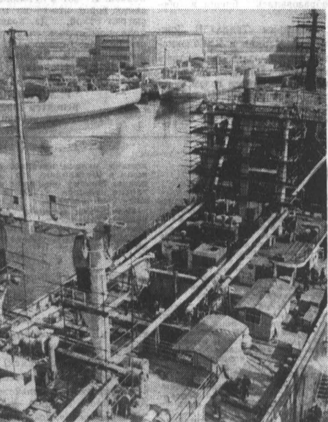
ПОЛЬША. Глянская верфь — одна из крупнейших в мире. Находясь в ознаменовании 50-летия Великого Октября присвоено имя Владимира Ильича Ленина. За два десятилетия с ее стальной плечи на воду 468 судов, из них 351 судно общего назначения и 1 миллион 637 тысяч тонн построено по заказам Советского Союза.
