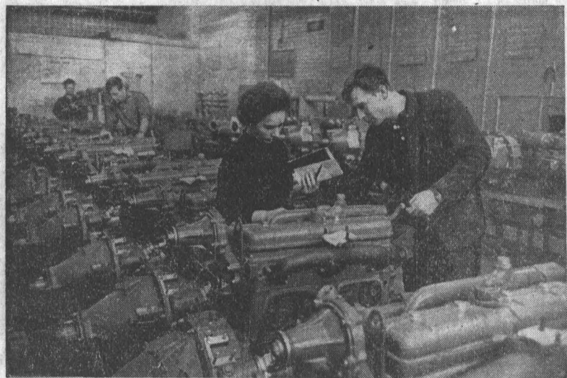
Алтайский тракторный завод. Участок экспортерной сборки двигателей «СМД-7» еще и в праздники Октябрь выполнил свое годовое задание. Сейчас коллектив этого участка ведет сборку двигателей для вьетнамских друзей. НА СНИМКЕ: на переднем плане старший мастер Б. И. Помилунов (справа) и контролер П. М. Антимонова. Фото В. Николаева.
