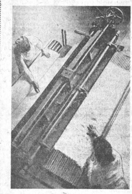
На снимке: изготовление мягких прошивных холстов из стекла. Фото Г. Никитина. Фотохроника ТАСС.
