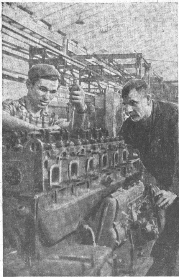
Собран и отправлен на АТЗ первый серийный двигатель АМ-01. НА СНИМКЕ: слесари-сборщики Валерий Кулинич (слева) и Виктор Богданов за изготовлением первого алтайского мотора мощностью 130 лошадиных сил. Фото В. Николаева.
