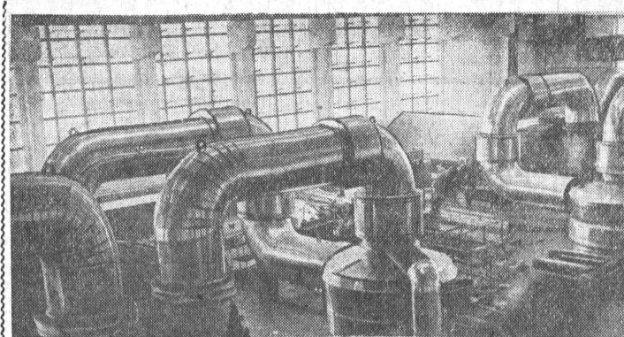
В разгаре строительство Нововоронежской атомной станции. В аппарате и турбинном залах идет монтаж оборудования. Электрики и специалисты по электронному прибору устанавливают и настраивают аппаратуру на главном щите управления. Велик объем работ на сооружении химической водоочистки. Эта сложная система предназначена для выделения радиоактивных остатков из воды, используемой при работе станции. Все вредные вещества будут подаваться в места,
