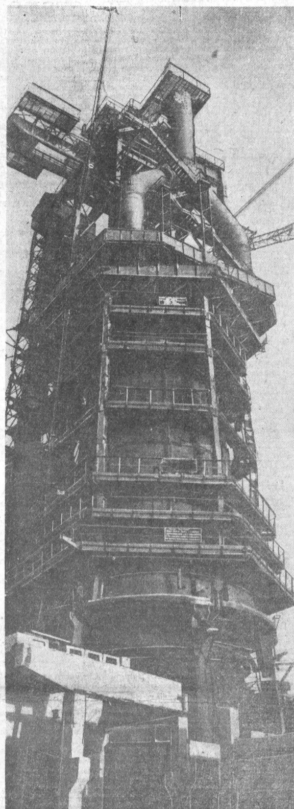
Казахская ССР. Быстрыми темпами возводится вторая домна Казахской Магнитки. Замечательна монтаж узлов колошников, пылеуловителя, скрубберов. Монтажные управления «Базальконструкция» установили купол последнего из четырех воздухоподогревателей печи. На снимке: строящаяся вторая домна Карагандинского металлургического завода. Фото Я. Турбина. Фотохроника ТАСС.
