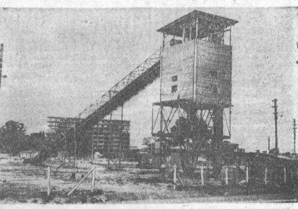
Турция. В пригороде Стамбула с помощью Советского Союза построен бетонный завод производительностью около 50 тысяч кубометров бетона в год. Предприятие оснащено новейшей советской техникой. Все производственные процессы механизированы и автоматизированы. На снимке: на бетонном заводе. Фото И. Угольнова. Фотохроника ТАСС.
