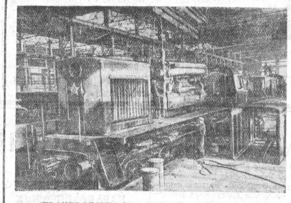
ПРОИЗВОДСТВО МАНЕВРОВЫХ ТЕПЛОВЗОВОВ. На Брянском машиностроительном заводе вступил в строй новый цех, выпускающий маневровые тепловозы мощностью 1000 лошадиных сил. Они предназначены для маневровых работ на железнодорожных узлах. Для производства тепловозов построены специальный корпус, оснащенный высокопроизводительным оборудованием. На снимке: сборка маневровых тепловозов. Фото И. Рабиновича. Фотохроника ТАСС.
