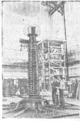
Москва. Производственные бригады завода «Изолятор» закончили сборку двух высоковольтных масляных трансформаторов на напряжение 500.000 вольт.
