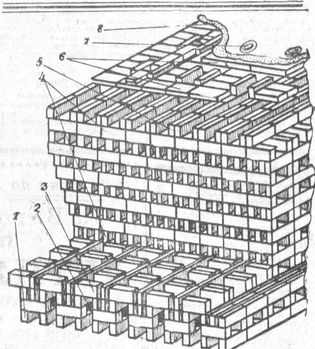
Черт. № 2. Схема садки кирпича: 1. «Ножки», 2. Подовый канал, 3. Перекрытие «ножки», 4. Елка (8—14 ряды), 5. Слово перекрытия, 6. Перекрытие садки, 7. Подовые конфорки, 8. Засыпка земли.
