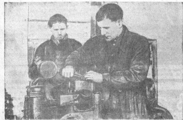
Отлично трудятся в честь выборов в Верховный Совет СССР механизаторы Мамонтовской МТС Н. Ковальчук и А. Шершнев. Нормы выработки они ежедневно перевыполняют в полтора раза. На снимке: Н. Ковальчук (справа) и А. Шершнев за сборкой мотора трактора ДТ-54.
