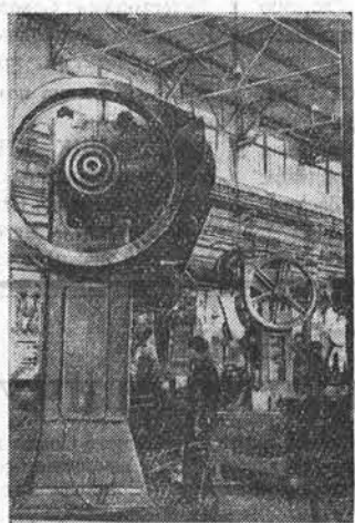
В прессовом цехе Алтайского тракторного завода виден комбинированный штамп, позволяющий за один ход ползуна пресса штамповать две детали. Металлическая лента подается для штамповки автоматическим. Такое мероприятие обеспечило значительное снижение себестоимости деталей и больше чем в два раза повысило производительность труда.
