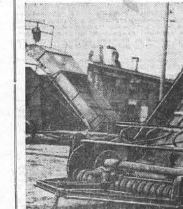
Аномалинс. Завод «Казаксельмаш» освоил производство новой сельскохозяйственной машины — подборщика-копнителя. Она состоит из трех основных узлов: подборщика, элеватора и копнителя. Во время движения машинист «гладит» подборщика подхватывают с земли скошенное сено и поддают его на переднюю часть элеватора. Транспорт элеватора передвигает сено в камеру копнителя. При заполнении камеры один из рабочих нажимает на педаль механизма сбрасывания, и копка падает на землю. Ширина захвата подборщика-копнителя два метра. За рабочий день новая машина собирает в копны сено с площади 70—80 гектаров. Обслуживают ее два человека. На снимке: внешний вид подборщика-копнителя. Фото А. Матвеева. (Фотокорреспондент ТАСС).
