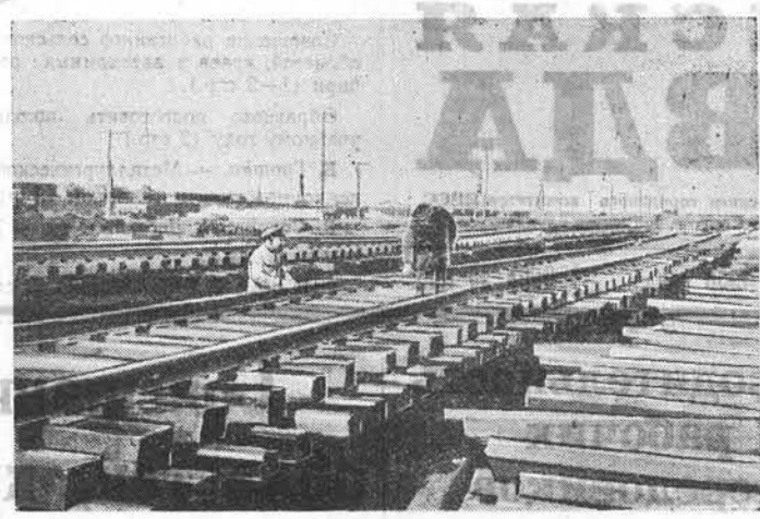
На строительстве железнодорожной линии Карасук—Камень. На снимке: звенооборочная база. Перед отправкой готовых звеньев пути на трассу. Фото В. Николаева.
