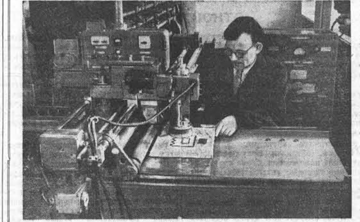
Москва. Во Всесоюзном научно-исследовательском институте автогенной обработки металлов разработана конструкция и изготовлен образец машины для лазерной резки металла «МДМ-2». Новая машина предназначена для вырезки деталей сложной конфигурации по чертуну-копиру или металлическому шаблону из листов толщиной до 200 миллиметров, шириной до 2,5 метра и длиной до 10 метров и более. Испытательная часть снабжена шестью резаками, что позволяет вырезать одновременно 6 одинаковых деталей и значительно повышает производительность. Помимо магнитно-копировального механизма имеется фотоинтерпретационное устройство, что делает возможным применение чертежей-копиров, выполненных на бумаге. Машина может производить масштабное копирование по чертуну или металлическому шаблону в масштабе до 1:10 (по отношению к размерам вырезаемой детали). Это позволяет снизить затраты на изготовление и хранения чертунной и шаблонной и сократить время, затрачиваемое на их установку и уборку. На снимке: ведущий конструктор машины Ю. В. Курлов подкладывает чертун-копир под фотоэлектрическую головку копировальной части машины «МДМ-2».
