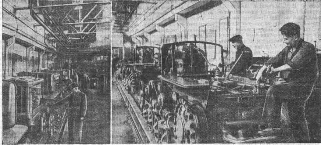
Общий вид главного конвейера.
