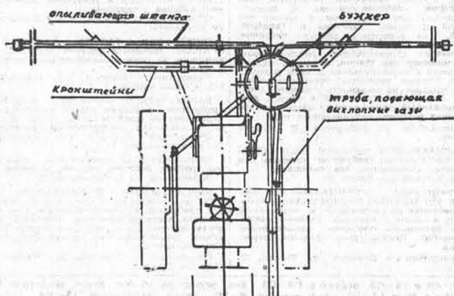
Схема оборудования опылывателя.
