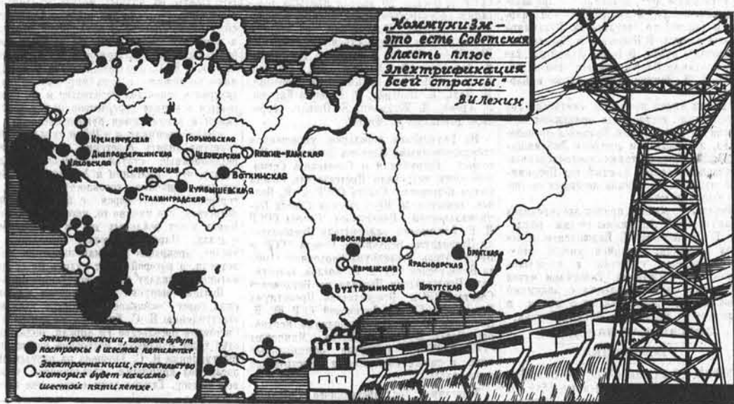
Карта расположения крупнейших электростанций, строительство которых будет завершено или начато в шестой пятилетке.
