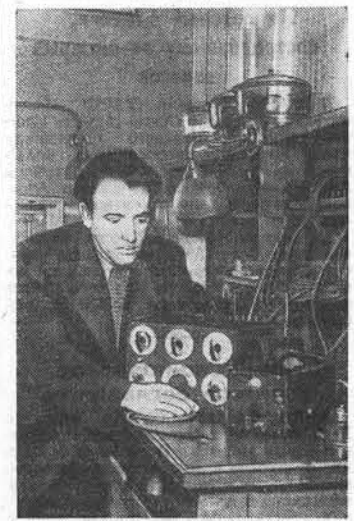
Ленинград. В агрофизическом научно-исследовательском институте успешно закончены испытания нового прибора. Он предназначен для измерения температуры и автоматической сигнализации при перегреве воздуха в зерносушилках, элеваторах, овоцехранилищах, силосных ямах, на складах угля. Автор этого изобретения — старший инженер-конструктор Б. М. Шлимович. Новый прибор измеряет температуру при помощи полупроводниковых термомостов. Автоматическое устройство обеспечивает поочередное подключение электротермометра к измерительному прибору. Если температура выше допустимой, то возникает звуковой и световой сигналы, указывается место перегрева. На снимке: старший инженер-конструктор Б. М. Шлимович за испытанием прибора. Фото И. Баранова. (Фотохроника ТАСС).
