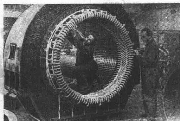
В Венгерской Народной Республике в минувшем году довоенный уровень промышленного производства превзойден в три с половиной раза. Уровень многих предприятий освоили выпуск сложных машин и станков. На снимке: обработка статора гидрогенератора в цехе завода имени Кlementa Готвальда в Будапеште. Фото Мадяр фото.
