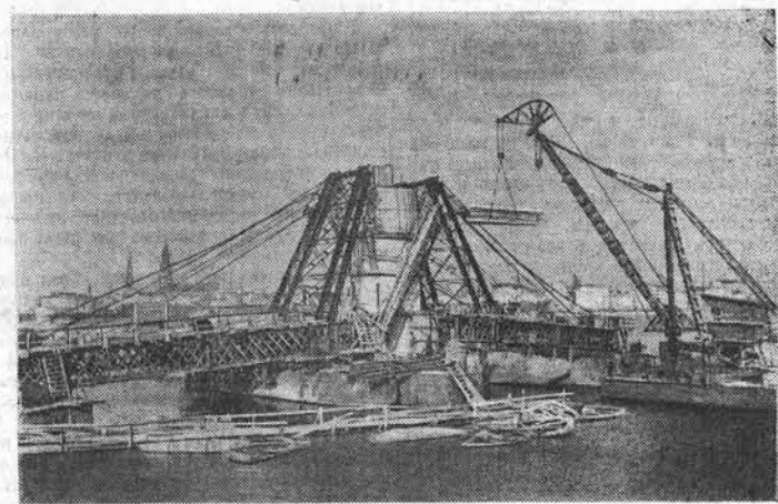
В Риге идет строительство большого автогужового моста через Даугаву. Он устанавливается на бетонных, облицованных гранитом опорах. Прозрачная часть моста будет достаточно широка, чтобы обеспечить интенсивное движение трамваев, автомашин и пешеходов. Два центральных пролета приспособляются для прохода под ними небольших судов. Для пропуска более крупных пароходов на правом берегу рени обустраивается подъемный пролет. С помощью специальных механизмов он будет подниматься вверх и оплыв устанавливаться на место. Огражденный красивыми металлическими перилами, мост перекрестит над водами Даугавы почти на километра в длину. НА СНИМКЕ: один из участков строительства. Фото Е. Ясенова. (Фотокроника ТАСС).
