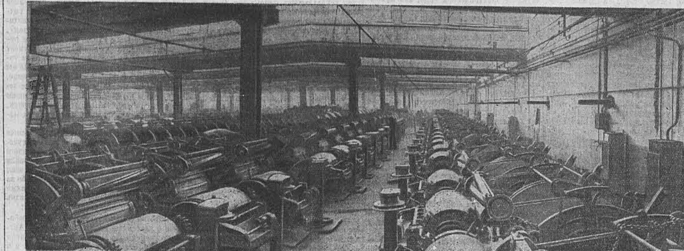
В Барнауле сооружается крупнейший в Сибири хлопчатобумажный комбинат. В эти дни в его цехах идет монтаж оборудования. В прядильной фабрике уже полностью установлены чесальные машины.
