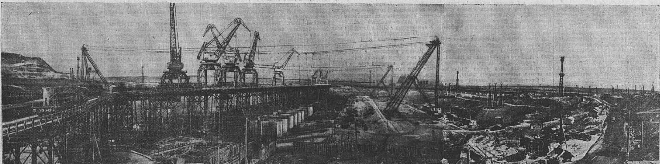
КУЙБЫШЕВГИДРОСТРОЙ. Общий вид строительства здания Куйбышевской ГЭС. Вдоль всего котлована идет бетоновозная эстакада.
