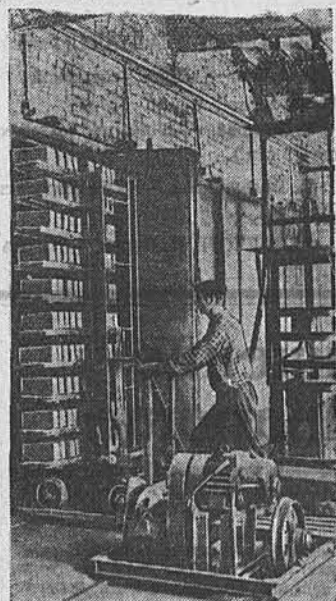
Трест «Стройгаз» заканчивает строительство нового завода кирпичного производства в 12 миллионов штук в год. Завод оборудован механизмами новой конструкции — вакуумпрессом, полуавтоматом для резки кирпича и сыра, электрокарами для загрузки и разгрузки сушильных камер. Сейчас ведутся работы по освоению отдельных участков завода. На снимке: момент загрузки сушильных камер кирпичом-сырцом. Фото Н. Калинин.
