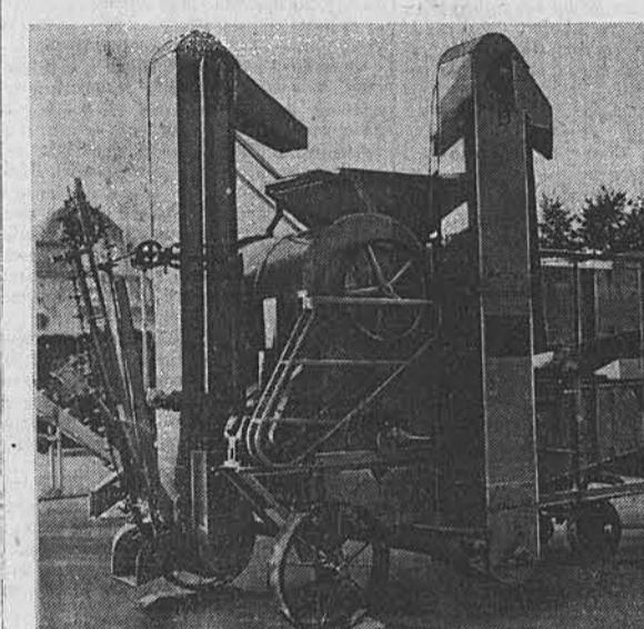
Новая зерноочистительная машина „ЗМК-2“ Челябинским тракторным заводом изготовлена новая зерноочистительная машина „ЗМК-2“ системы работника Увельского зерносовхоза Челябинской области А. А. Кузнецова. Новая машина предназначена для очистки различных сельскохозяйственных культур — пшеницы, ржи, овса и других — до степени продовольственного зерна высокого качества. В отличие от других зерноочистительных машин подобного типа «ЗМК-2» имеет следующие эксплуатационные особенности: высокую производительность — до 15 тонн в час на пшенице, механизированную подачу зерна в бункер и механизированную выгрузку очищенного зерна в автомашину. В действие машина приводится от электромотора мощностью 4,5 киловатта. Вес ее 1.710 килограммов. На снимке: новая зерноочистительная машина «ЗМК-2» на Всесоюзной сельскохозяйственной выставке. Фото Л. Портера. (Фотохроника ТАСС).
