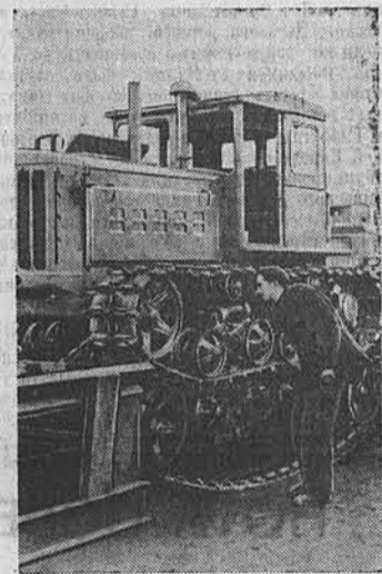
Участник предоктябрьского социалистического соревнования — регулировщик тракторосборочного цеха Алтайского тракторного завода Н. Воронков четко ведет регулировку и испытание трактора. На снимке: Н. Воронков у испытательного стенда. Фото А. Калабухова.
